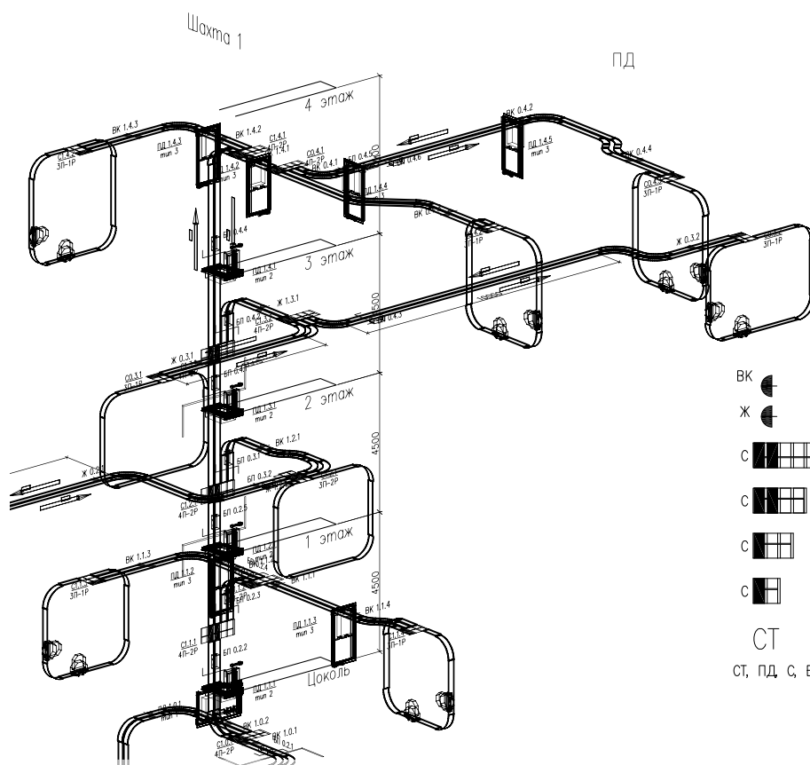
Изометрическая схема монорельсовой транспортной системы адресной доставки изданий для Азербайджанской национальной библиотеки
